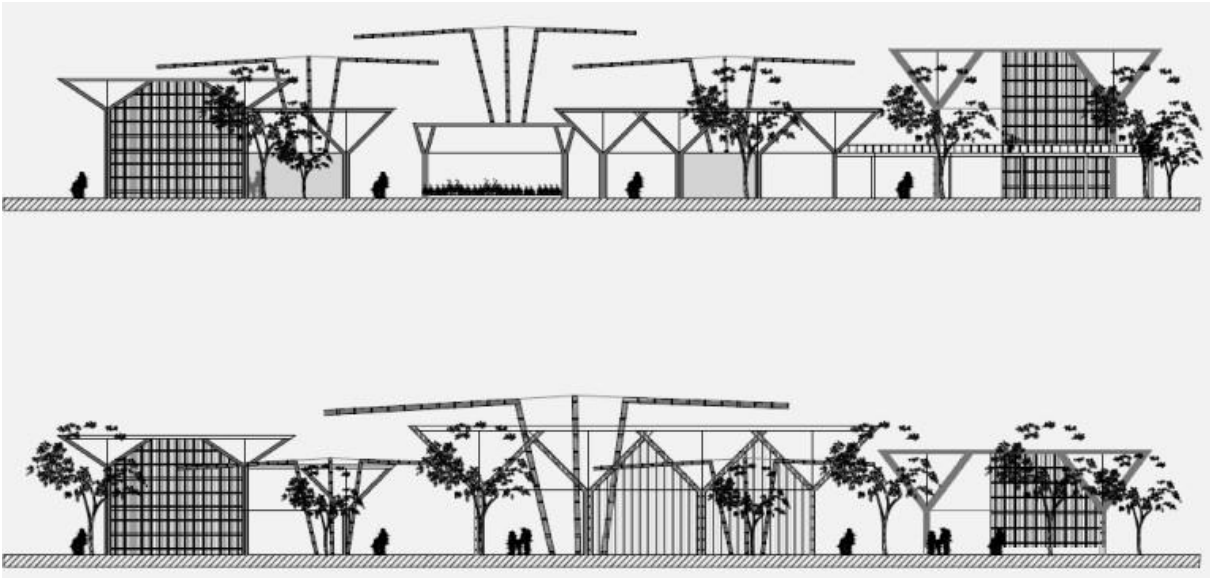
Figura 33. Fachadas arquitectónicas. Fuente propia (2019).
