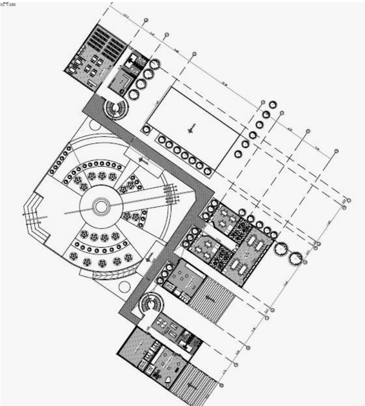
Figura 32. Planta nivel 2. Fuente propia (2019).
